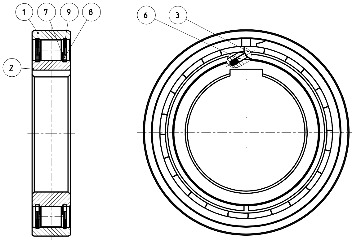
Abb.1 Aufbau Freilaufkupplung AE
