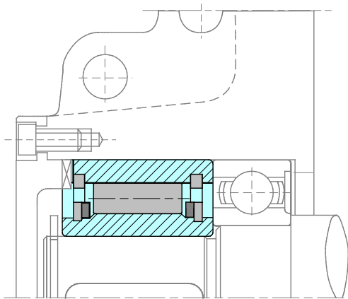
Abb. 3: Einbaubeispiel AE
