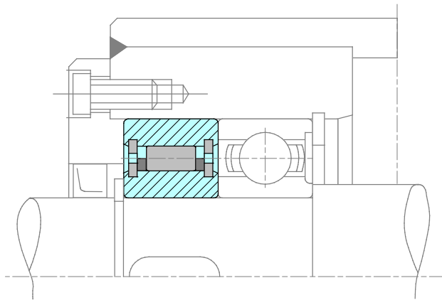
Abb. 3: Einbaubeispiel AS
