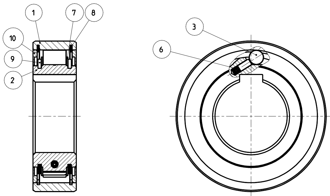
Abb.1a Aufbau Freilaufkupplung AS
