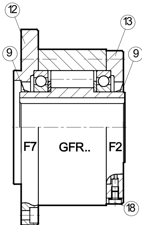
Abb.1c Aufbau GFR..F2F7
